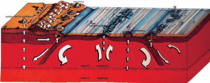
ESQUEMA DE LOS TIPOS DE MÁRGENES DE PLACAS Y SU MOVIMIENTO
